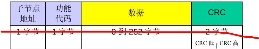
图 9: RTU 报文帧
