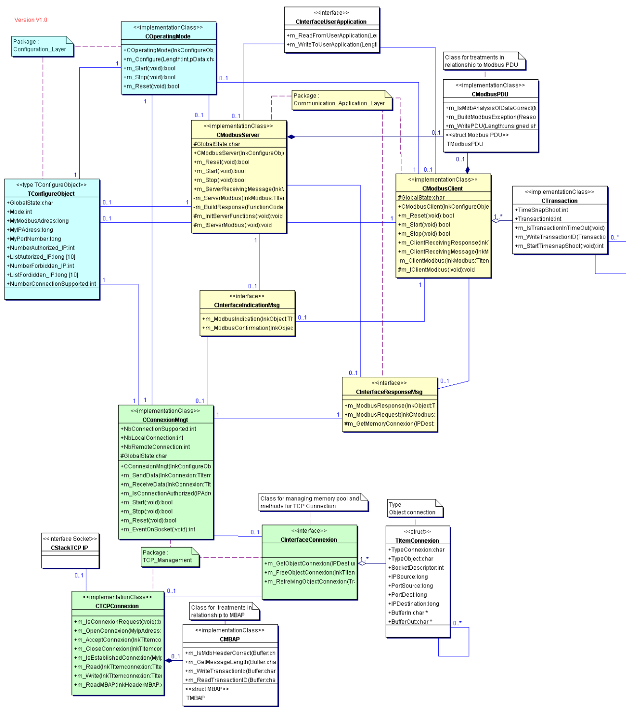
图 22：类的示意图
